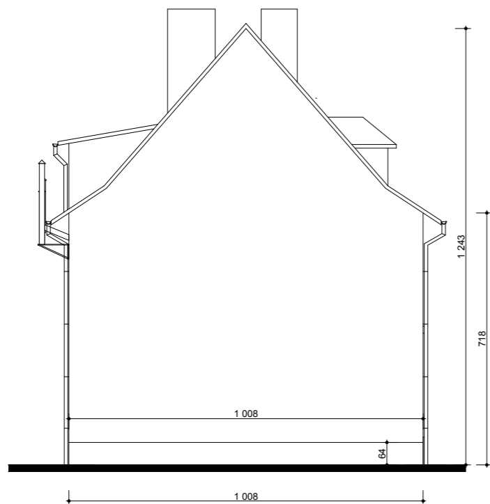
ELEWACJA BOCZNA
