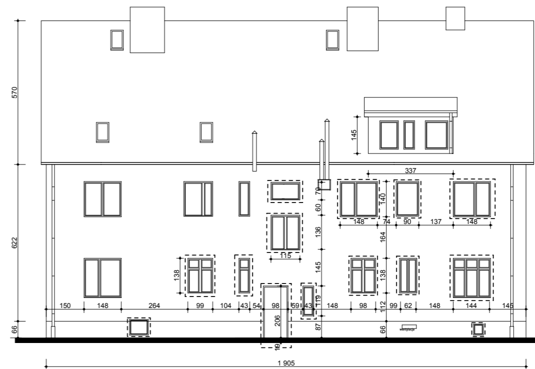
ELEWACJA TYLNA
