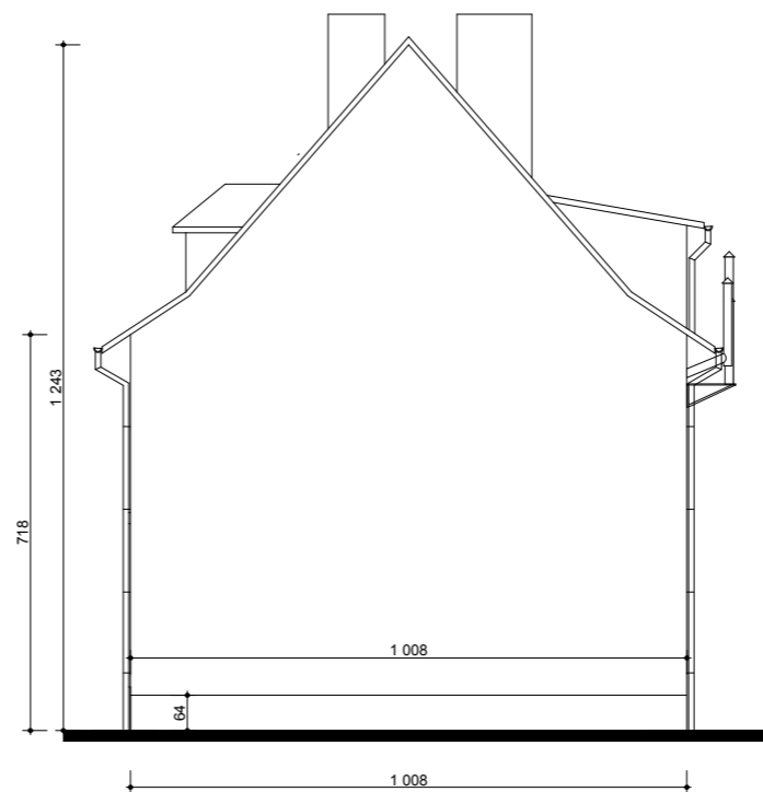
ELEWACJA BOCZNA
