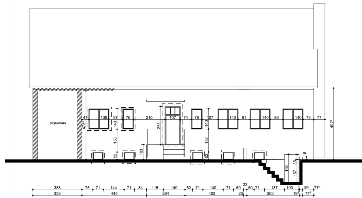
ELEWACJA TYLNA
