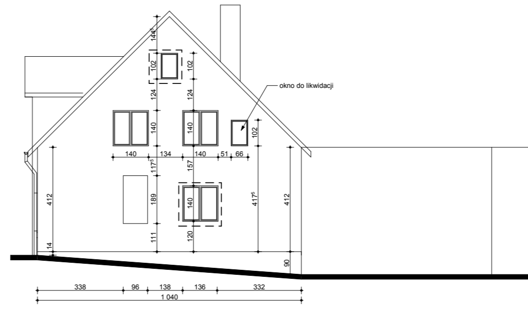
ELEWACJA BOCZNA
