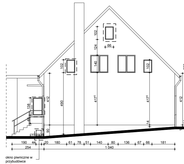
ELEWACJA BOCZNA
