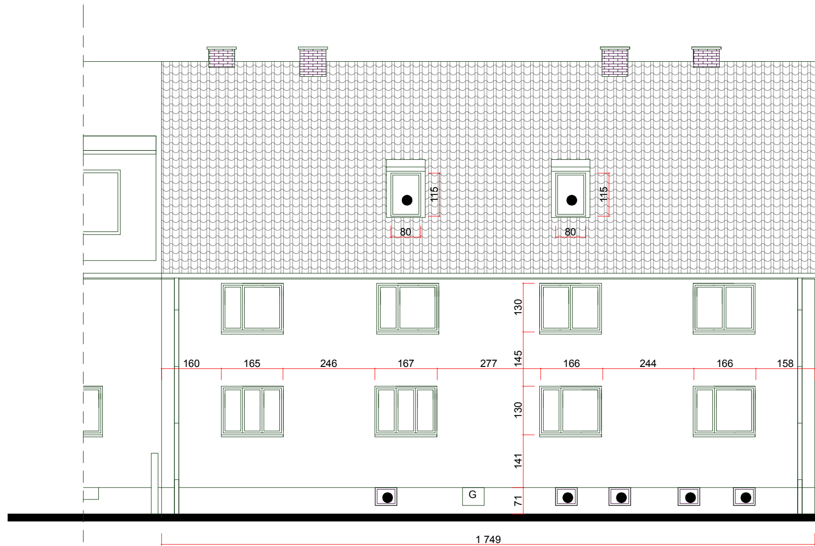
ELEWACJA FRONTOWA
