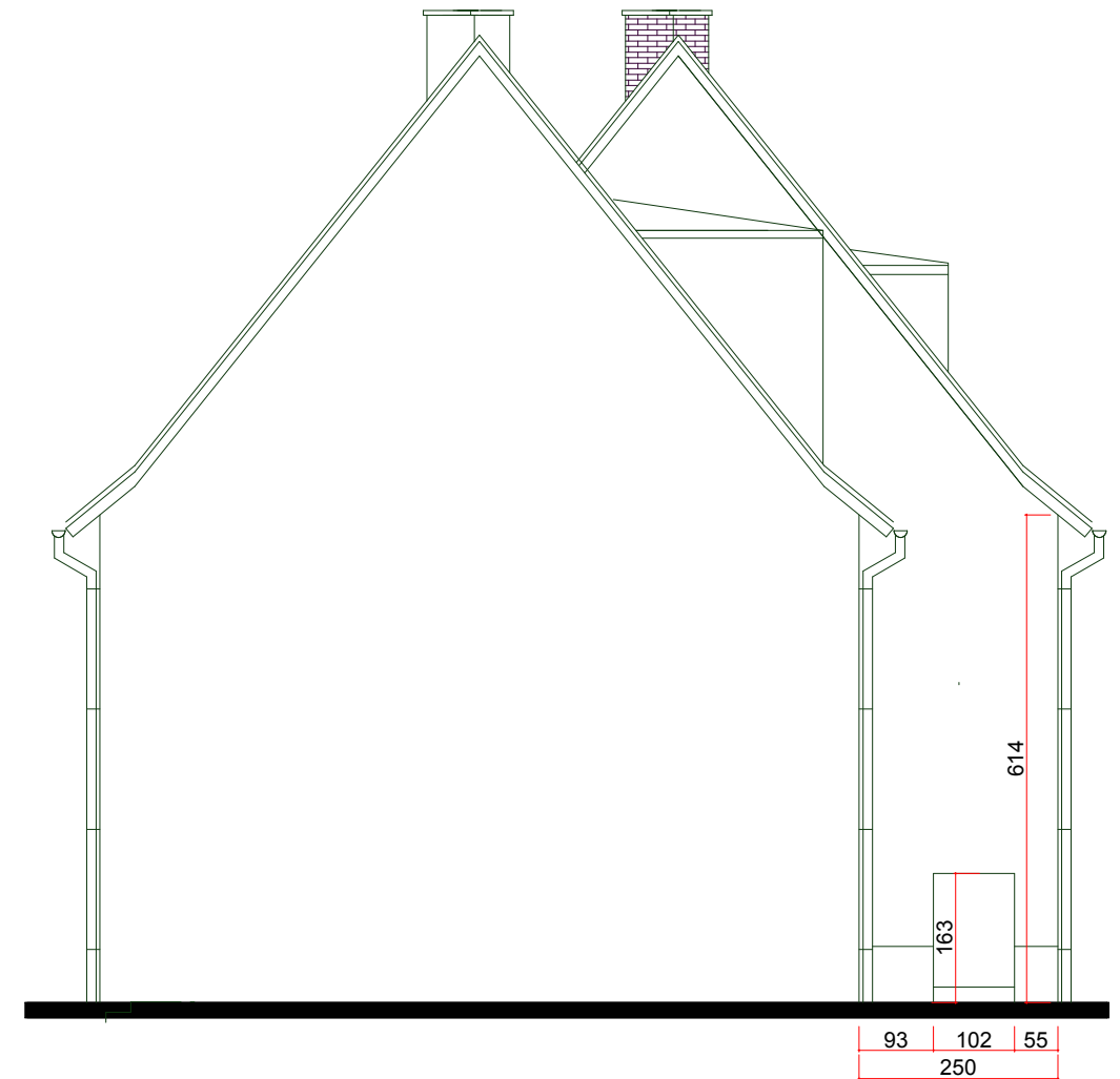
ELEWACJA BOCZNA
