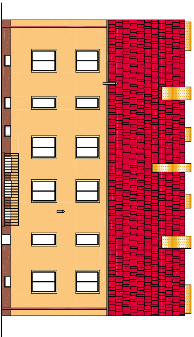
ELEWACJA ZACHODNIA
