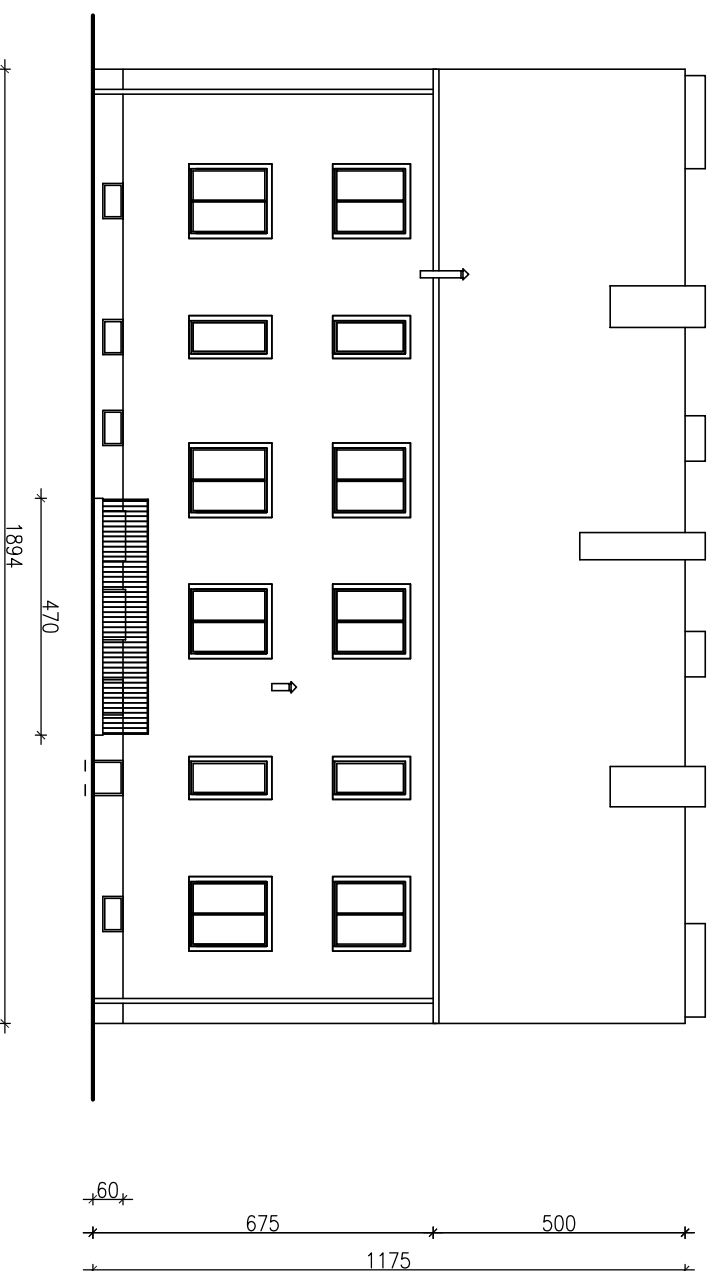
ELEWACJA ZACHODNIA
