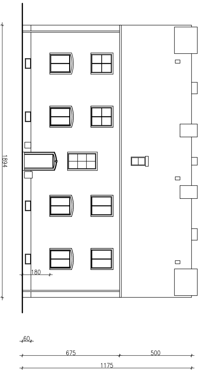
ELEWACJA WSCHODNIA
