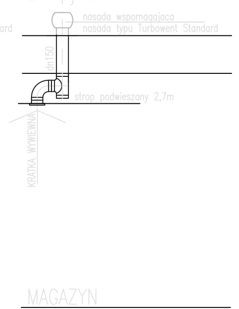
Przekrój C-C
