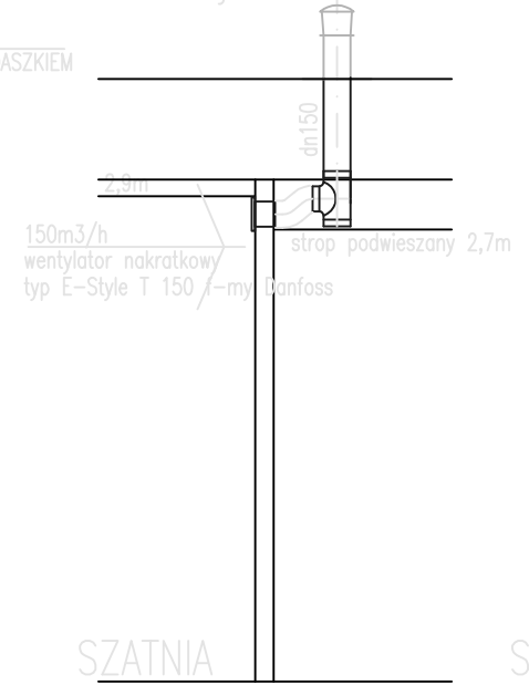
Przekrój A-A
