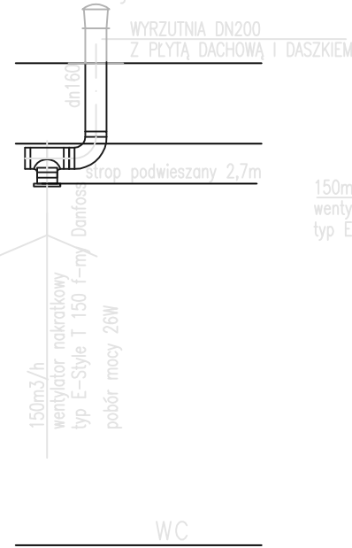
Przekrój E-E
