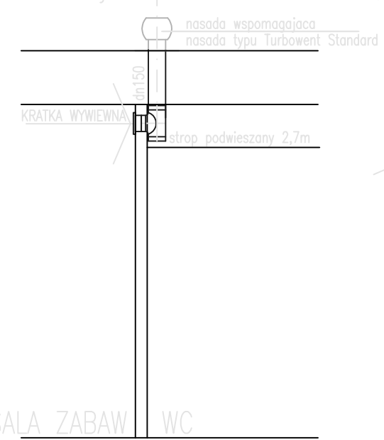
Przekrój B-B
