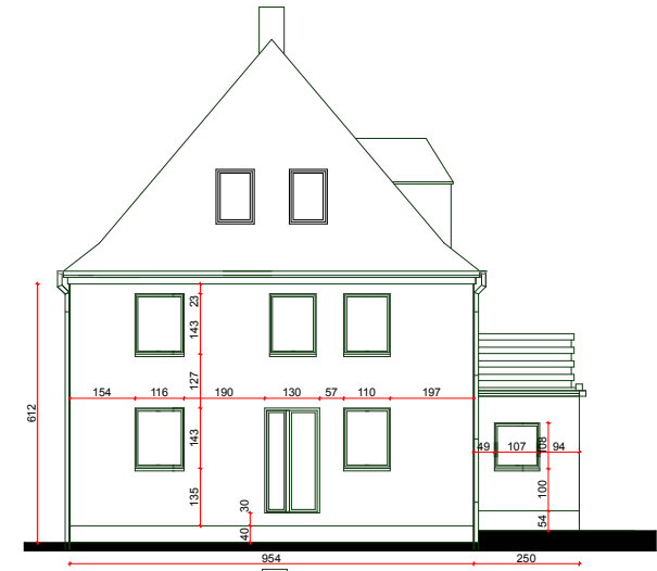
ELEWACJA BOCZNA
