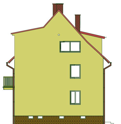
ELEWACJA BOCZNA
