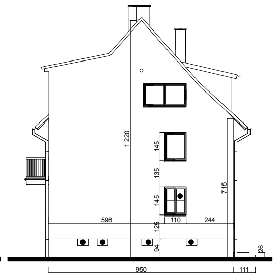
ELEWACJA BOCZNA
