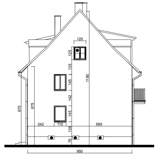
ELEWACJA BOCZNA
