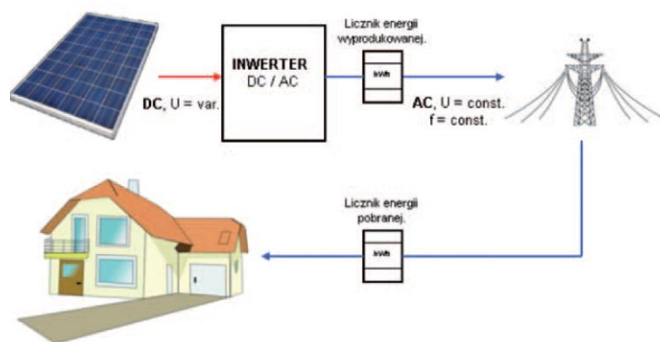
Rysunek 23. Schemat instalacji ON-GRID 174 (oznaczenia: DC- prąd stały, AC-prąd przemienny, U- napięcie, f-częstotliwość, var.-zmiennie, const.- stałe)
