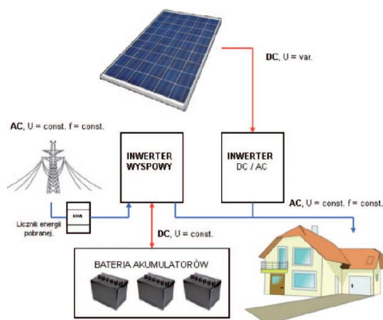
Rysunek 25 Schemat instalacji mieszanej 176 (oznaczenia: DC- prąd stały, AC-prąd przemienny, U- napięcie, f-częstotliwość, var.-zmienne, const.- stałe)
