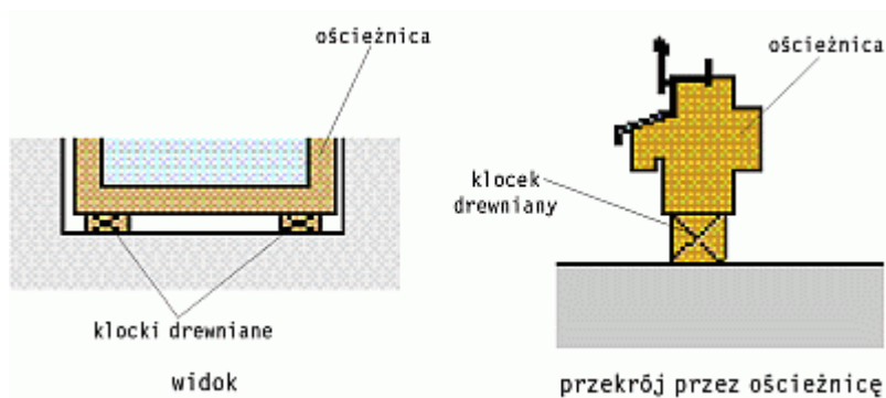
Podparcie na klockach progu ościeżnicy drewnianej okna jednoramowego
