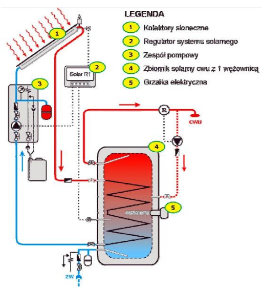
Rysunek 16. Schemat typowej instalacji słonecznej do podgrzewania ciepłej wody użytkowej 160
