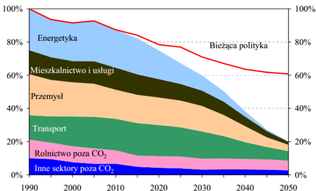
Rysunek 4. Mapa drogowa do niskoemisyjnej gospodarki. Redukcje emisji gazów cieplarnianych w poszczególnych sektorach 51
