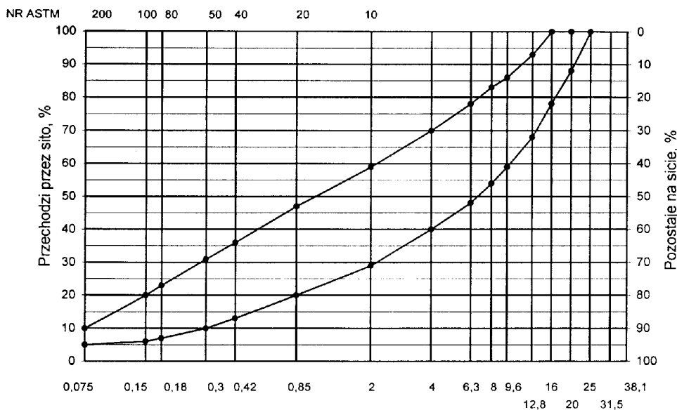
Rys. 1. Krzywe graniczne uziarnienia
