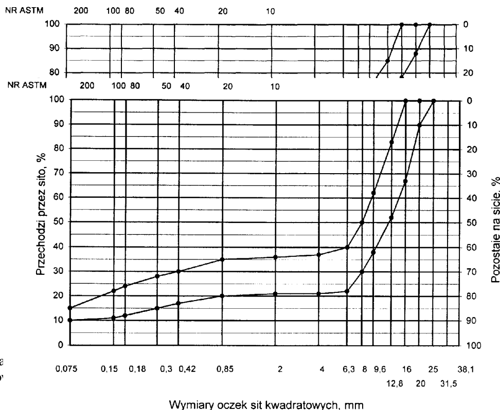
Rys. 4. Krzywe graniczne uziarnienia mieszanki mineralnej BA od 0 do 20 mm do warstwy ścieralnej nawierzchni drogi o obciążeniu ruchem od KR3 do KR6
