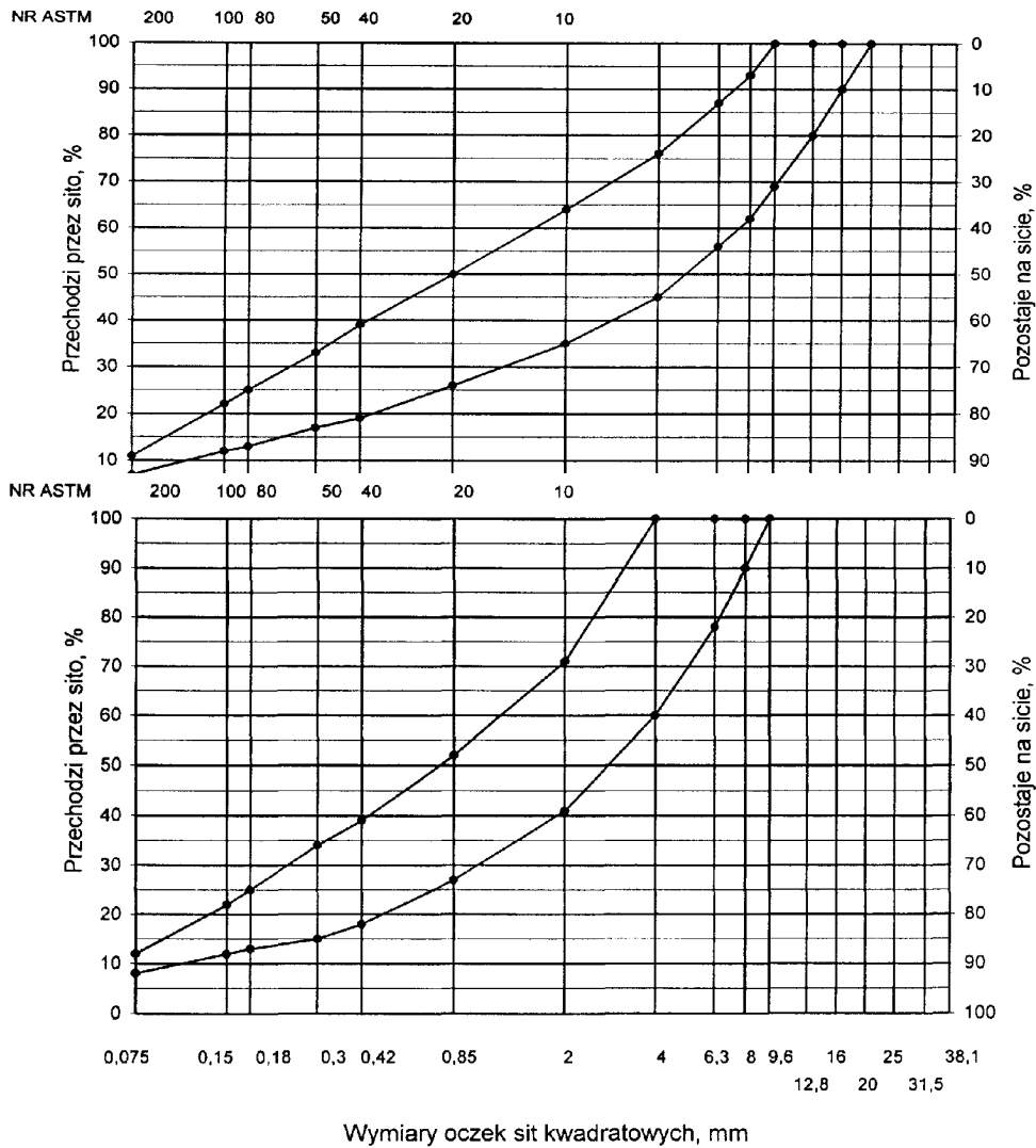
Rys. 2. Krzywe graniczne uziarnienia mieszanki mineralnej BA od 0 do 16mm, od 0 do 12,8 mm do warstwy ścieralnej nawierzchni drogi o obciążeniu ruchem KR1 lub KR2
