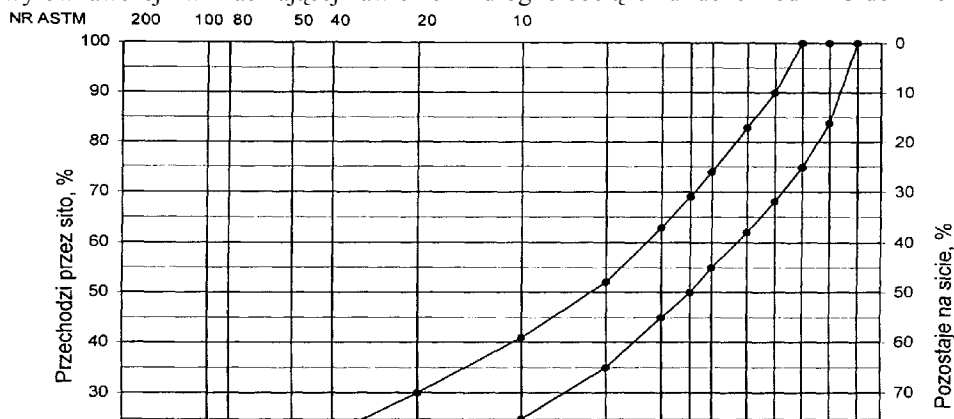
Rys. 12. Krzywe graniczne uziarnienia mieszanki mineralnej BA od 0
